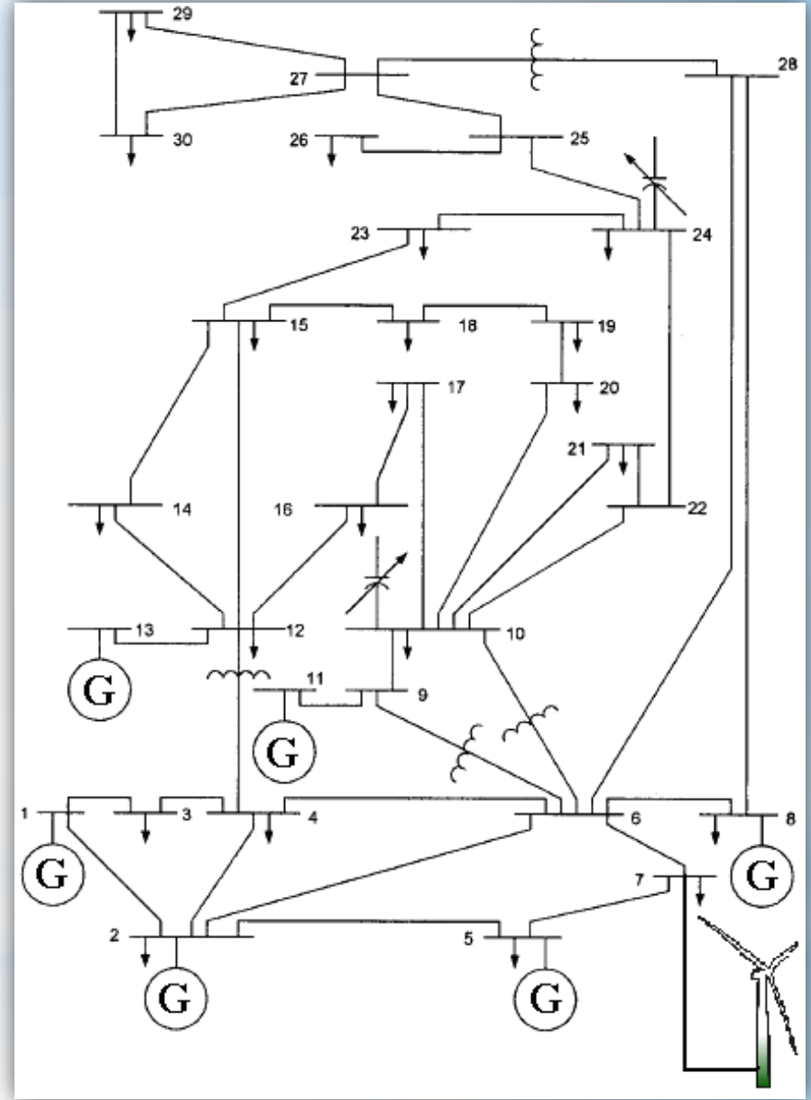
Resim 1. IEEE-30 baralı test sistemine eklenen rüzgar çiftliği
