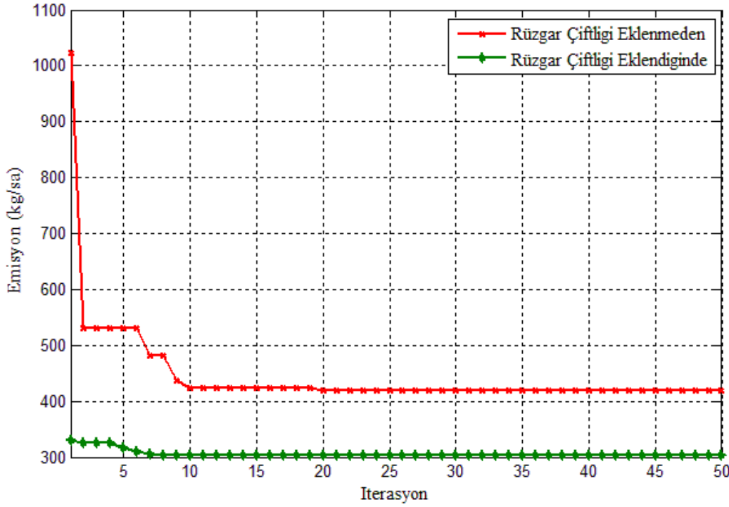
Şekil 2. Talep edilen 200 MW güç için rüzgar çiftliği eklenmeden ve eklendikten sonra oluşan emisyon eğrisi
