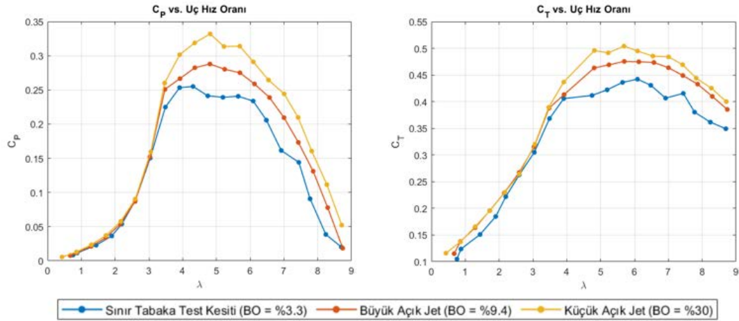
Şekil 10. Boyutsuz itki ve güç katsayıları (Merkez tüp kullanılarak elde edilmiştir)
