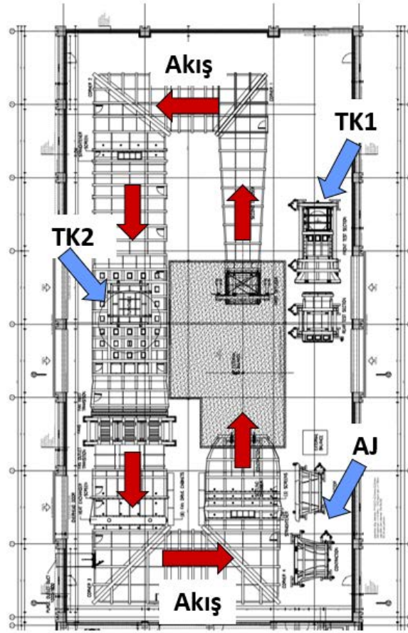
Şekil 3. ODTÜ-RÜZGEM BRT akış şeması (tünel içerisindeki akış doğrultusu kırmızı oklarla ifade edilmiştir)
