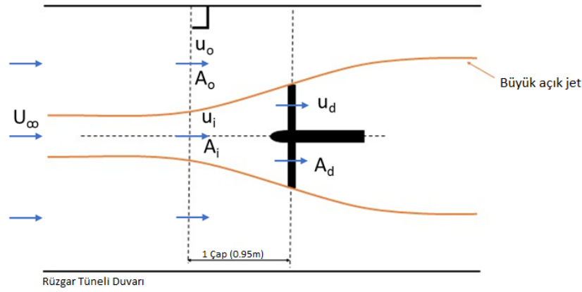
Şekil 9. Model rüzgar türbini üzerindeki akış şeması
