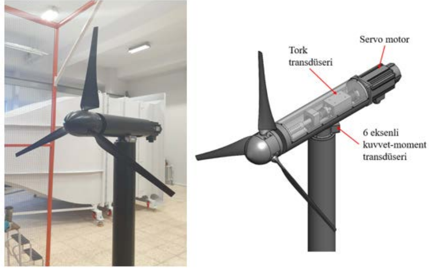
Şekil 5. Model rüzgar türbini
