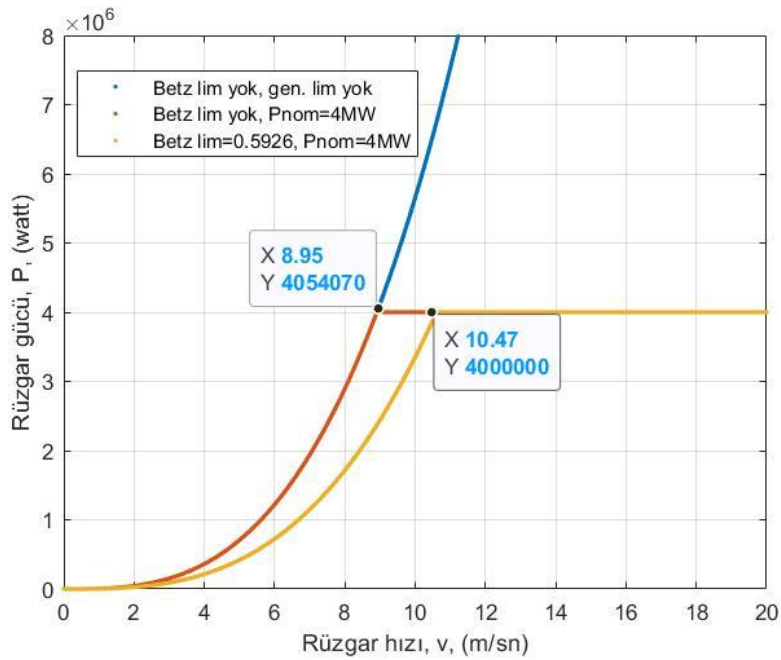
Şekil 2. Betz yasası ile rüzgâr hızına göre rüzgâr gücünün değişimi.
