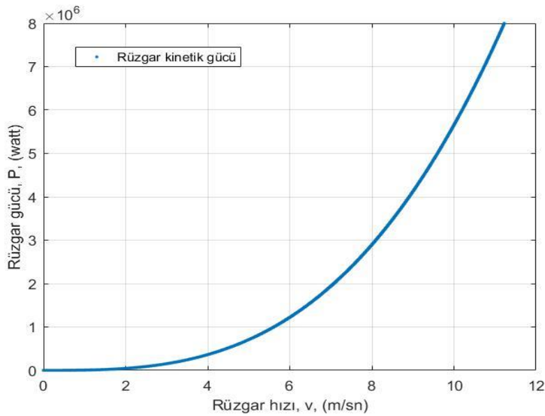
Şekil 1. Rüzgâr hızına göre rüzgâr gücünün değişimi.
