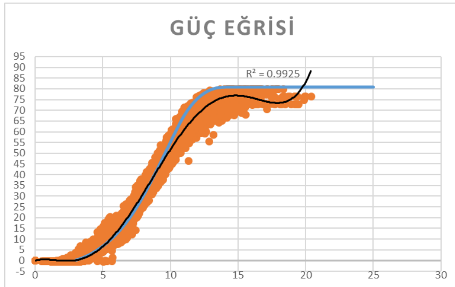
Şekil 6 Santral Güç Eğrisi
