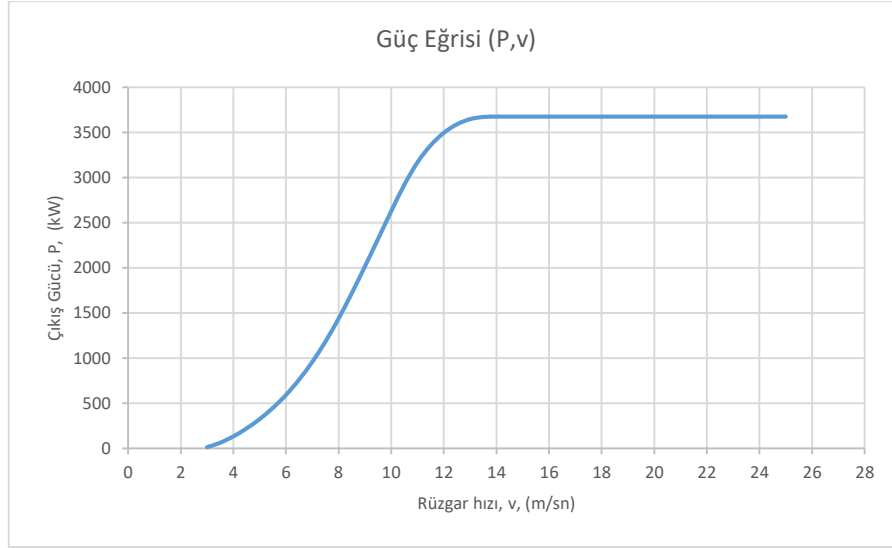
Şekil-4 Rüzgâr Türbini Güç Eğrisi
