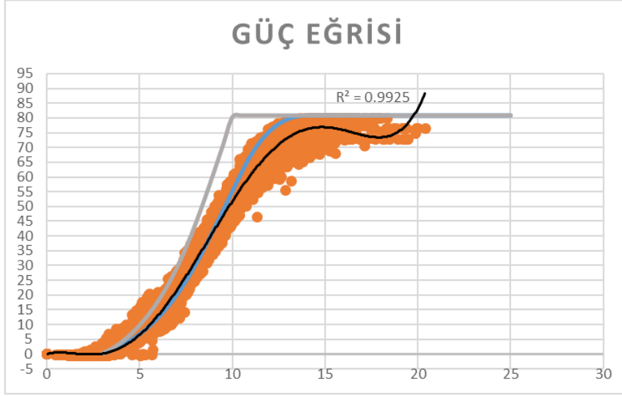
Şekil 7 Güç Eğrisi Dikleşmiş Santral Güç Eğrisi
