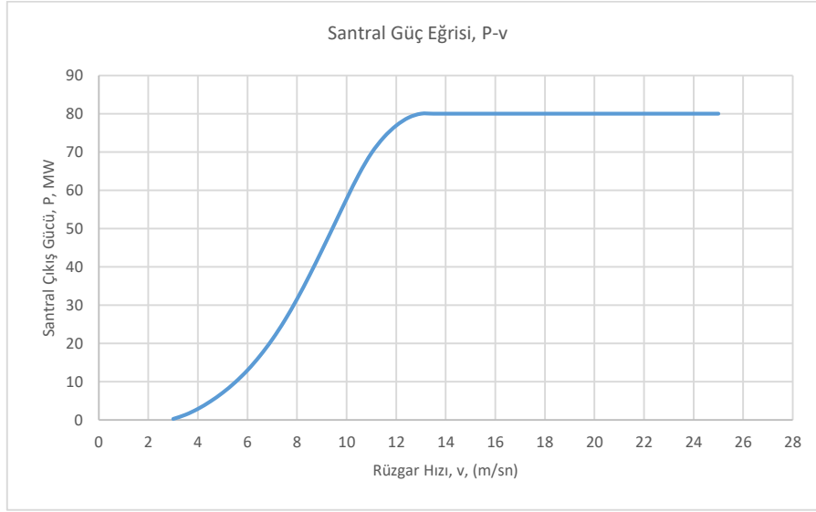
Şekil-5 Rüzgâr Santrali Güç Eğrisi
